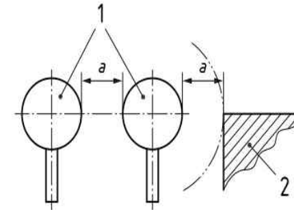
1 수동조작장치, 2 인접부품, a 최소거리
