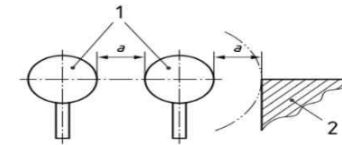
1 수동조작장치, 2 인접부품, a 최소거리
