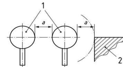
1 수동조작장치, 2 인접부품, a 최소거리
