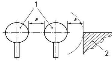
1 수동조작장치, 2 인접부품, a 최소거리
