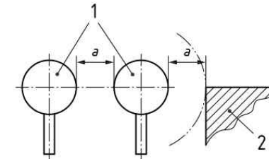
1 수동조작장치, 2 인접부품, a 최소거리
