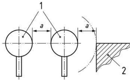
1 수동조작장치, 2 인접부품, a 최소거리
