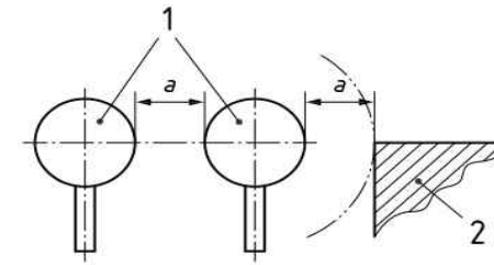
1 수동조작장치, 2 인접부품, a 최소거리
