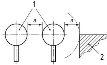
1 수동조작장치, 2 인접부품, a 최소거리
