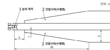
<그림 1 간접시야 영역>
