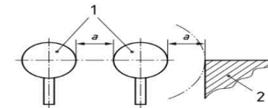
1 수동조작장치, 2 인접부품, a 최소거리
