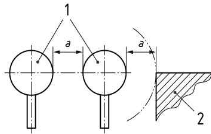
1 수동조작장치, 2 인접부품, a 최소거리
