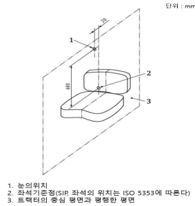
<그림 2 눈의 위치 세부 >
